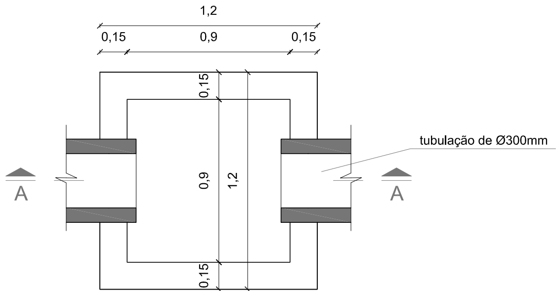
PLANTA BAIXA
