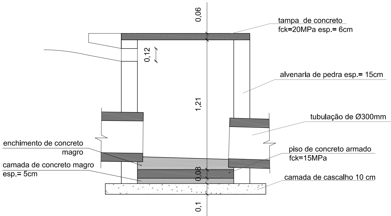
CORTE AA
