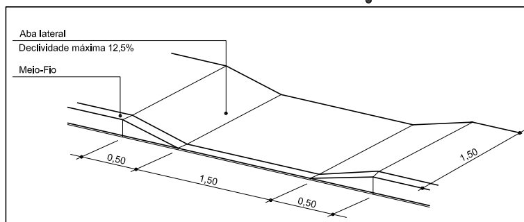
RAMPA DE ACESSIBILIDADE
