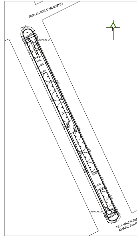
PLANTA BAIXA - ACADEMIA DE RUA COTADA AVENIDA TIRADENTES
