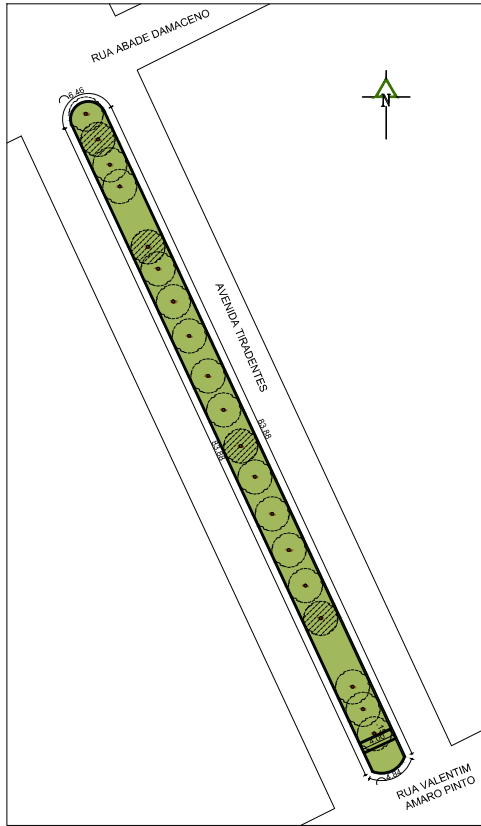
PLANTA BAIXA - EXISTENTE COTADA AVENIDA TIRADENTES
