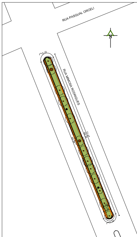
PLANTA BAIXA - EXISTENTE COTADA RUA MIMOSA RODRIGUES TRECHO 01
