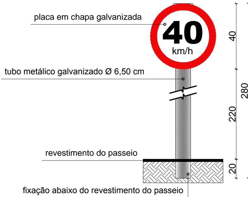
Suporte das Placas de Trânsito (medidas em cm)
