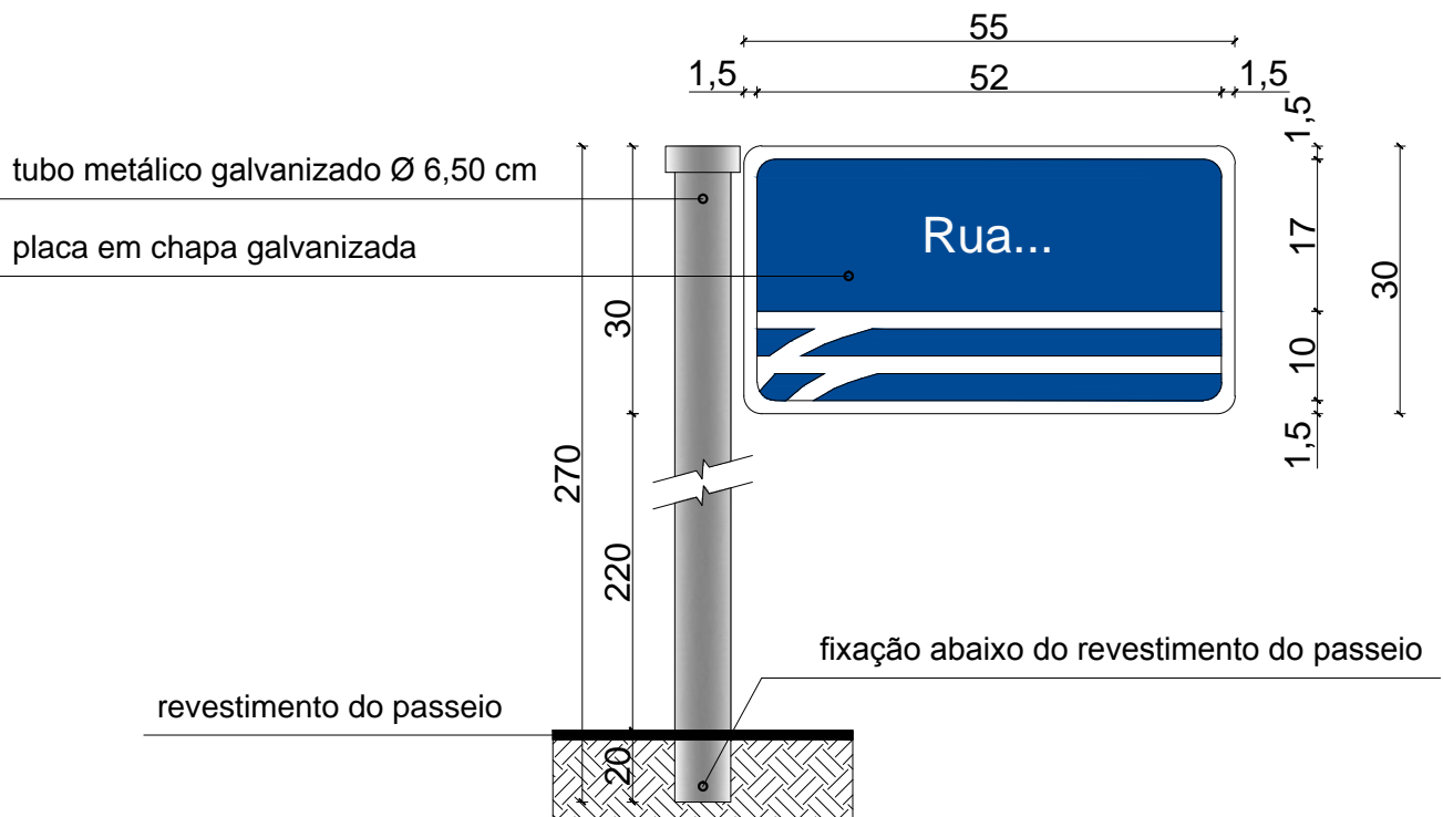
Placas 01, 02, 03, 04, 05 e 06 - Indicação de Ruas (medidas em cm)
